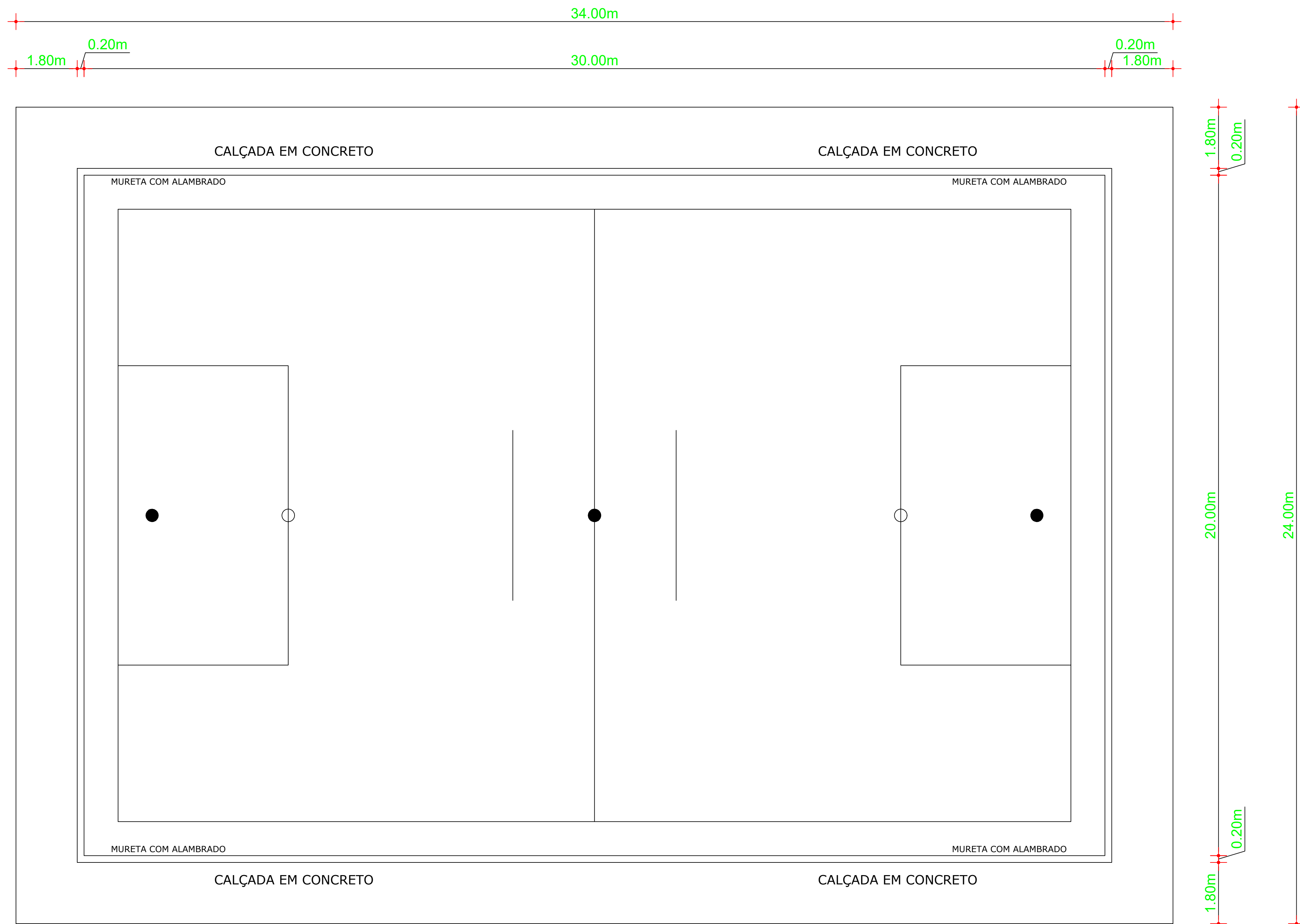
PLANTA BAIXA
