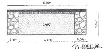
7 CORTE CC SEM ESCALA
