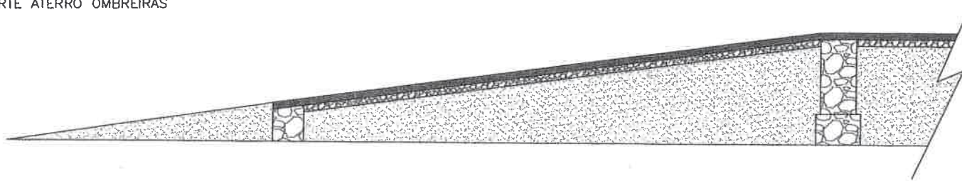
CORTE TRANSVERSAL
