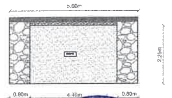
8 CORTE DD SEM ESCALA
