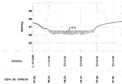
Perfil Longitudinal - PM
