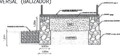
CORTE TRANSVERSAL (BALIZADOR)
