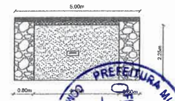
7 CORTE CC SEM ESCALA
