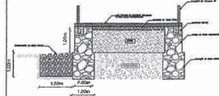
CORTE TRANSVERSAL (BALIZADOR)
