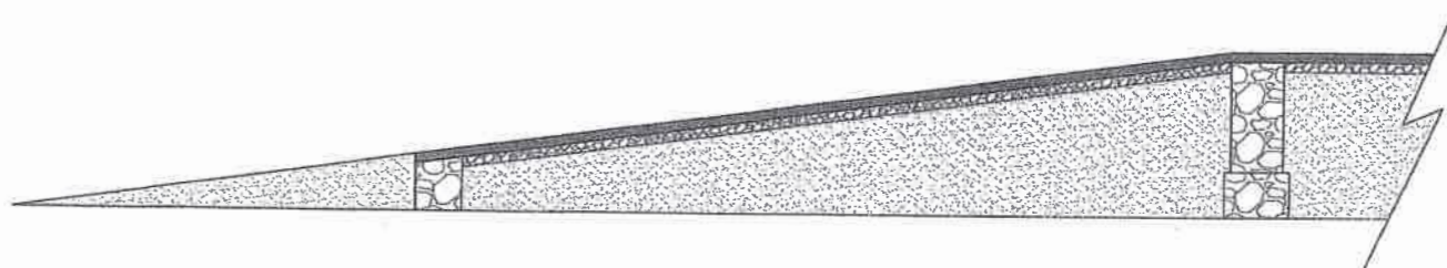
CORTE ATERRO OMBREIRAS
