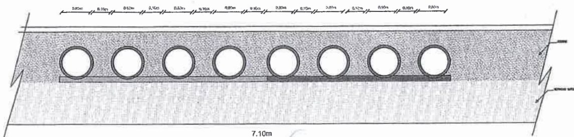
VISTA CORTE (DETALHE BUEIROS)
