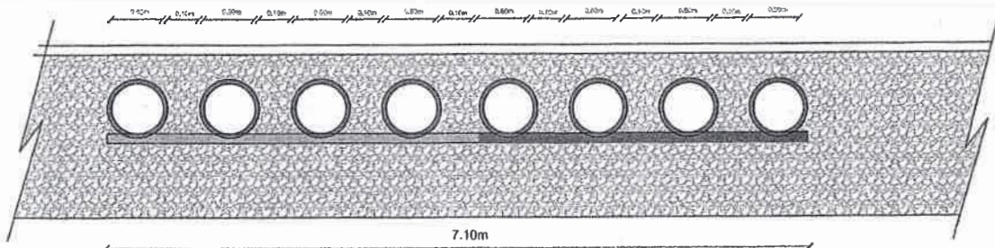
VISTA CORTE (DETALHE BUEIROS)
