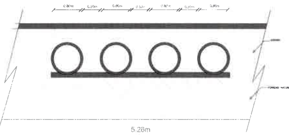
VISTA CORTE (DETALHE BUEIROS)
