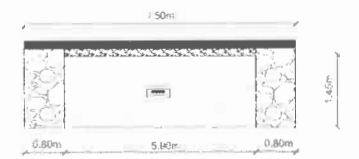
7 CORTE CC SEM ESCALA
