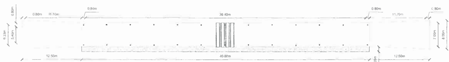
4 PLANTA BAIXA SEM ESCALA
