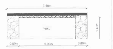
7 CORTE CC SEM ESCALA
