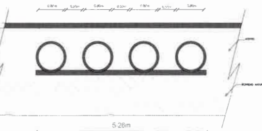
VISTA CORTE (DETALHE BUEIROS)
