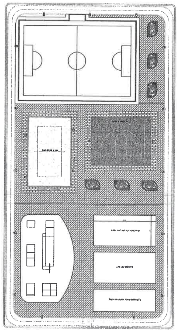
PLANTA PAGINAÇÃO
