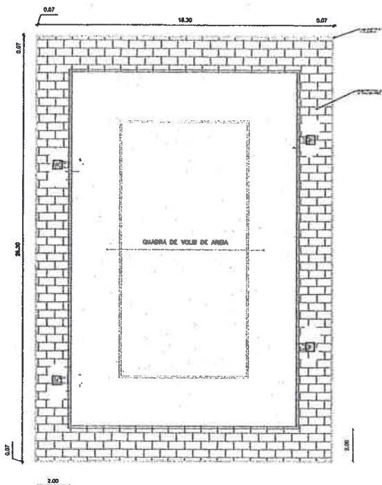
PLANTA PAGINAÇÃO
