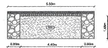
7 CORTE CC SEM ESCALA
