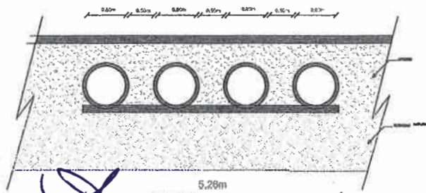
VISTA CORTE (DETALHE BUEIROS)
