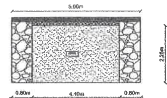
8 CORTE DD SEM ESCALA
