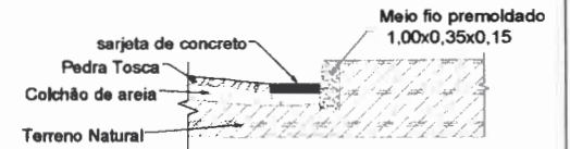
DETALHE SARJETA SEM ESCALA
