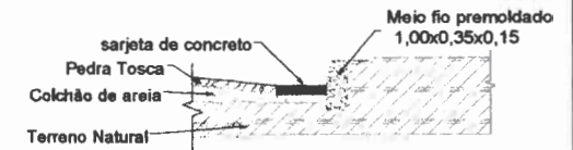
DETALHE SARJETA SEM ESCALA
